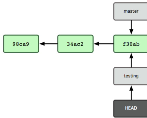
图 3.6: HEAD 在你转换分支时指向新的分支
