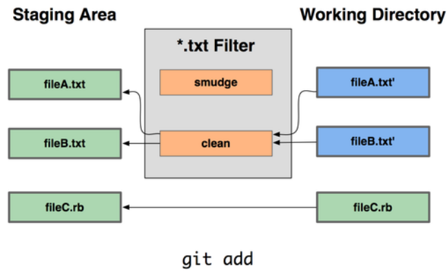
图 7.3: 提交到暂存区时, “clean” 过滤器被触发。
