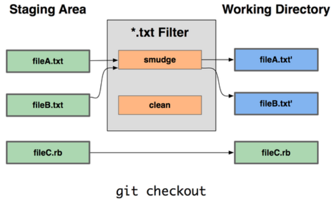
图 7.2: 签出时, “smudge” 过滤器被触发。
