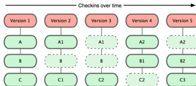
图 1.5: Git 保存每次更新时的文件快照
