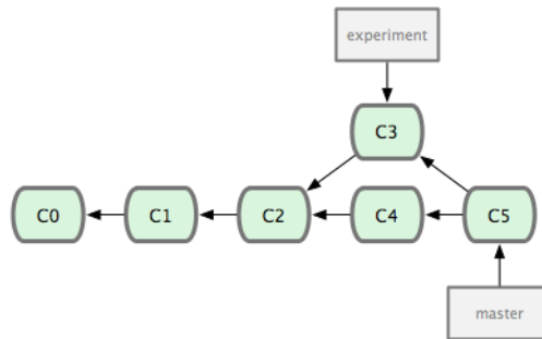
图 3.28: 通过合并一个分支来整合分支了的历史。
