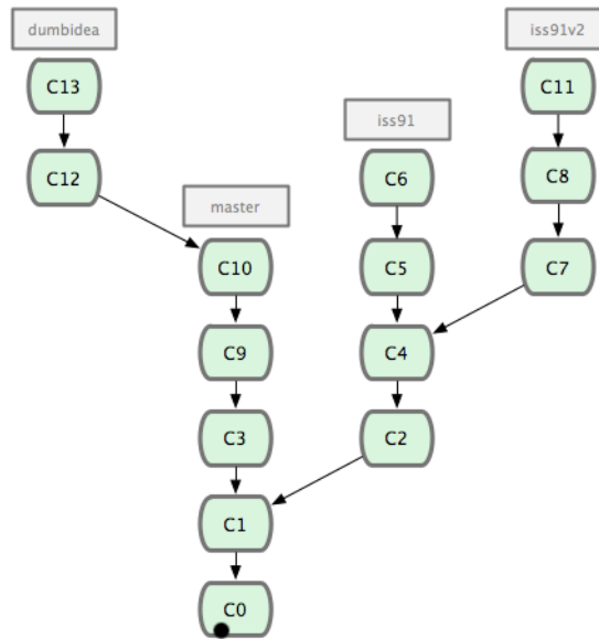
图 3.20: 拥有多个特性分支的提交历史。
