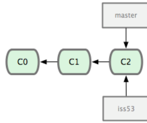
图 3.11: 创建了一个新分支的指针
