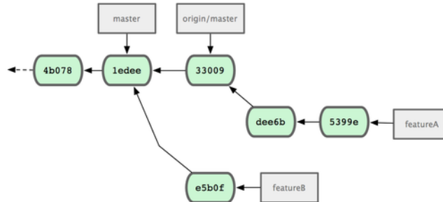
图 5.17: featureA 重新衍合后的提交历史
